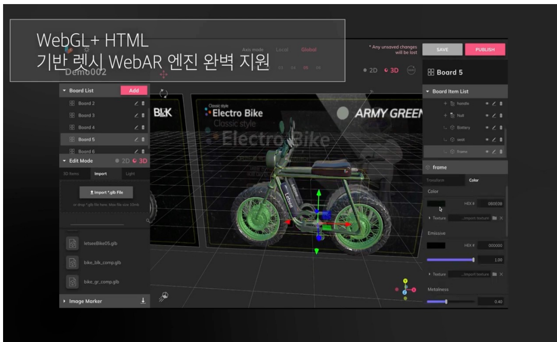
웹 기반 WYSIWYG 형식의 AR 콘텐츠 저작도구
